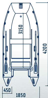
Solar-420 Strannik (Optima)
