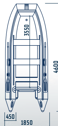
Solar-460 Strannik (Maxima)
