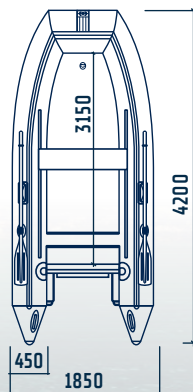
Solar-420 Strannik (Maxima)
